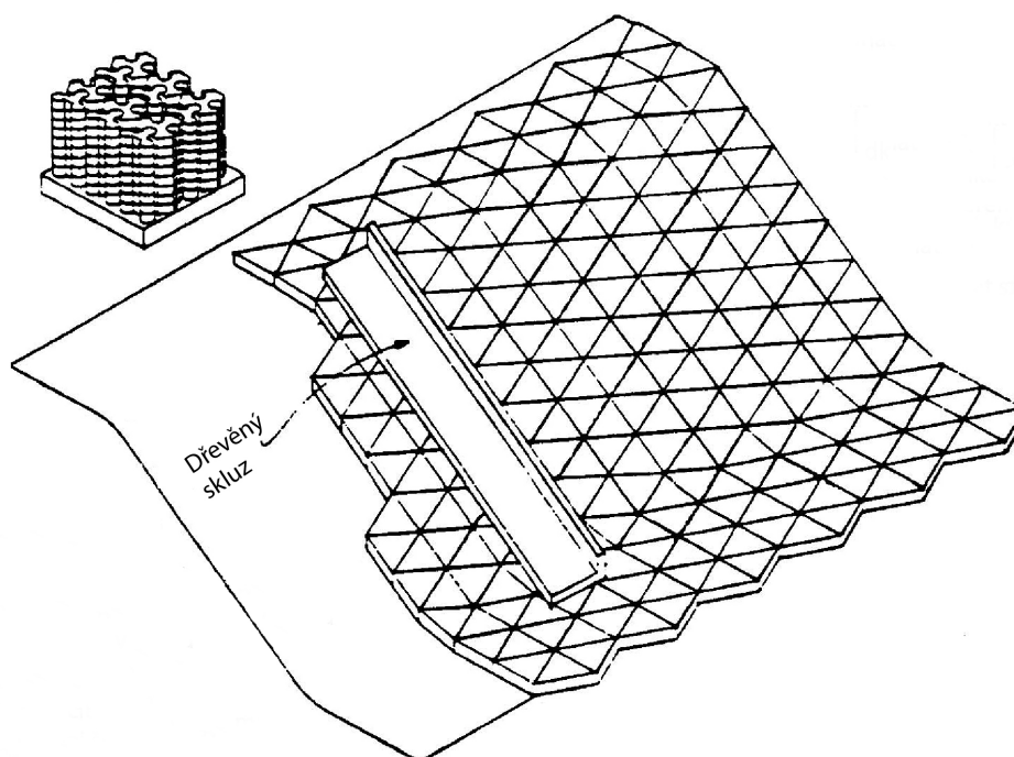
Obr. 3.3c Schematický pohled
